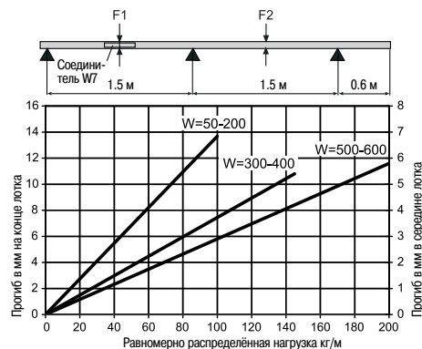
Расстояние между опорами (пролёт) - 2 м
