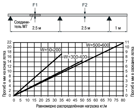
Расстояние между опорами (пролёт) - 2.5 м
