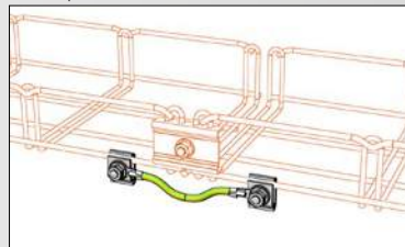
демонстрация монтажа
