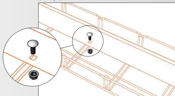
демонстрация монтажа
