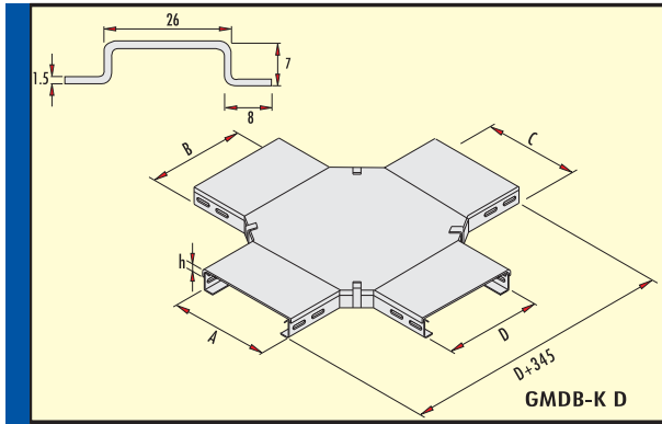
Dörtlü Bağlantı Eleman Kapağı Crossing Element Cover Пересечение Элемента Покрывтия
