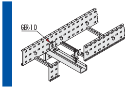
Merdiven Duvara ve Konsola Tespit Elemanı Ladder Fixing unit For Wall and Bracket
