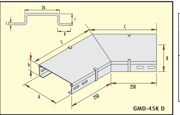
135° Dönüş Eleman Kapağı 135° Flat Bend Element Cover 135° Квартир Сгибают Элемент Покрывтия
