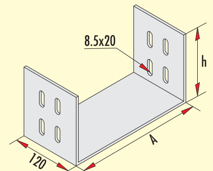
GTEP-C PG
