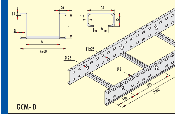
Ağır Hizmet Tipi Kablo Merdiveni (h=100 mm) Heavy Duty Type Cable Ladder (h=100 mm) Сверхмощные лестничные лотки
