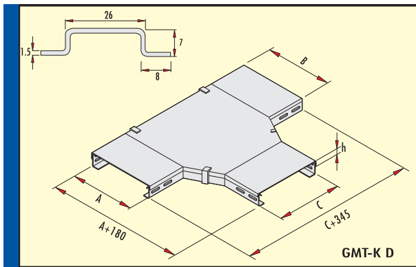
"T" Bağlantı Eleman Kapağı Tee "T" Element Cover Мишень "Т" Квартир Сгибают Элемент Покрывтия
