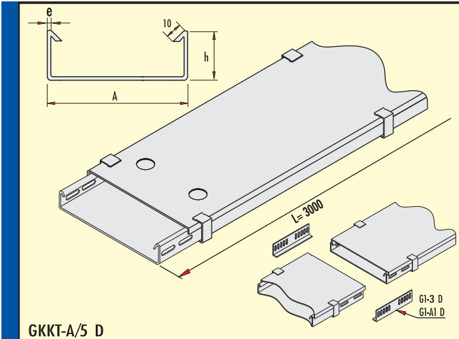
GKKT-A/5 D
