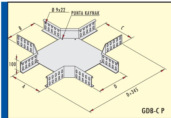
Ağır Hizmet Dörtlü Bağlantı Elemanı h=100 mm PASLANMAZ SAC (Cr-Ni) Heavy Duty Crossing h=100 mm Stainless Steel (Cr-Ni)
