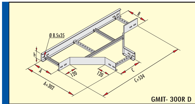
GMIT- D
