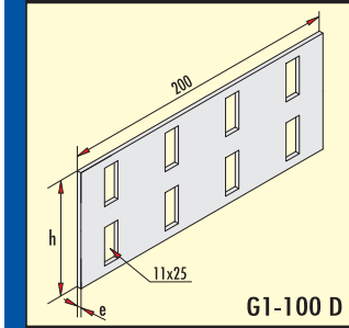
Ek Parçası Jointing Piece
