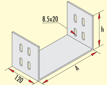
GTEP-B PG
