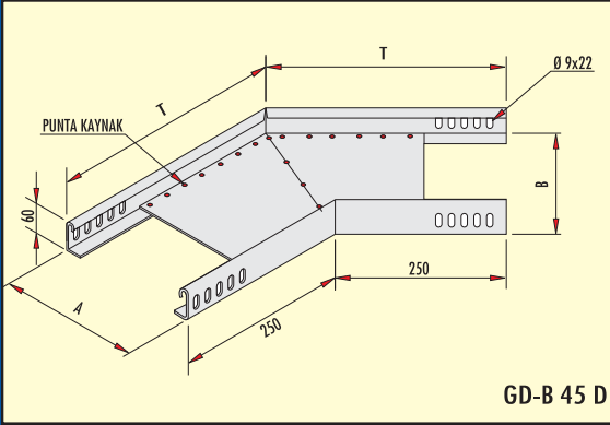
135° Ağır Hizmet Dönüş Elemanı (h=60 mm) 135° Heavy Duty Flat Bend (h=60 mm)
