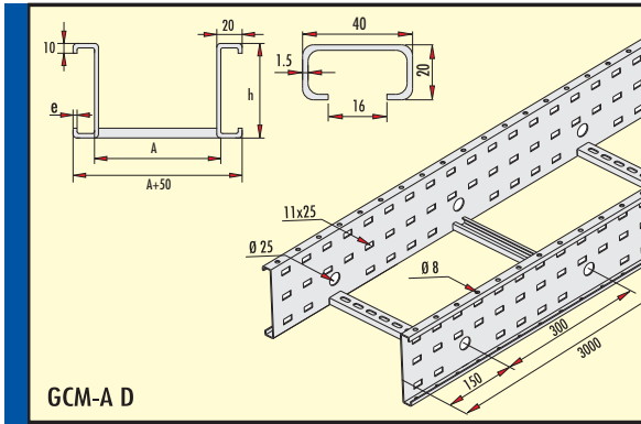
Ağır Hizmet Tipi Kablo Merdiveni (h=150 mm) Heavy Duty Type Cable Ladder (h=150 mm) Сверхмощные лестничные лотки
