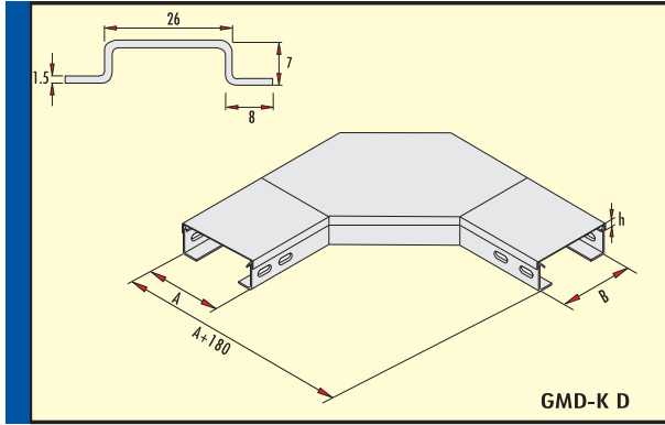
90° Dönüş Eleman Kapağı 90° Flat Bend Element Cover 90° Квартир Сгибают Элемент Покрывтия
