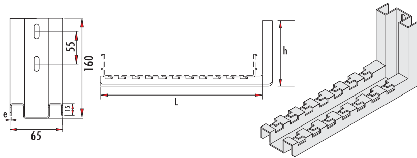
Tel Kanal Konsolu Wire-mesh bracket
