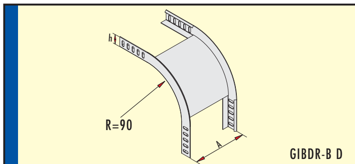
GIBR-B D
