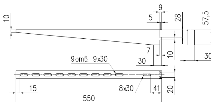
Полка кронштейна ПК 500 замковая
