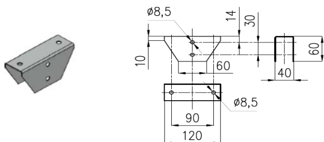
Элемент крепления к потолку сдвоенный КЭП 2
