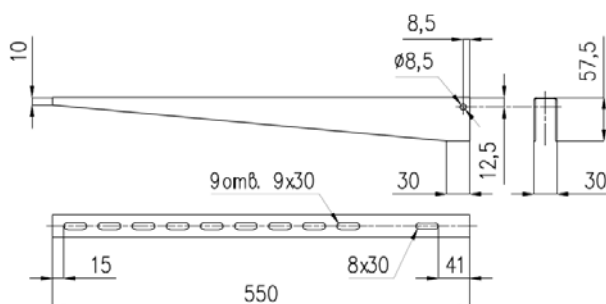
Полка кронштейна КП 500
