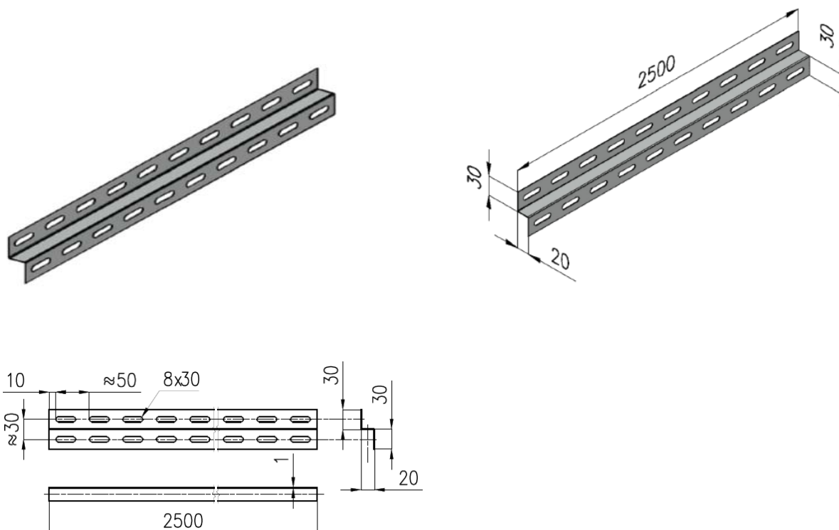
Z-профиль ZП
