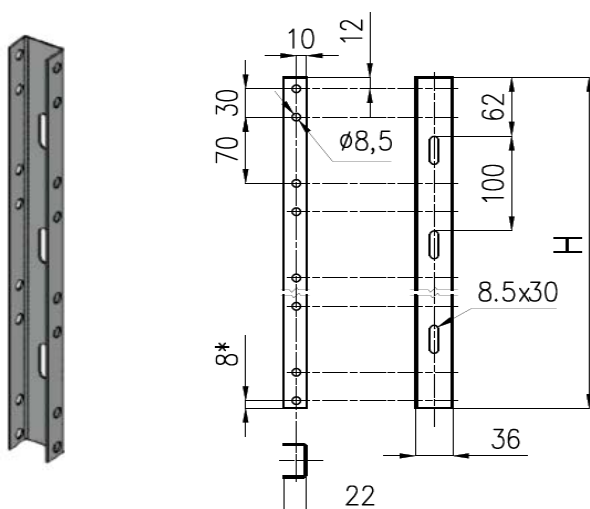
Элемент крепления к потолку КЭП
