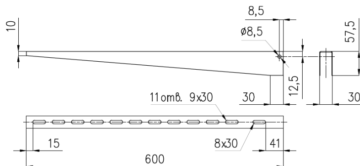
Полка кронштейна КП 600
