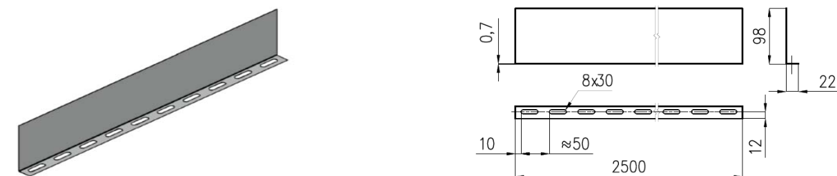
L-профиль ЛП 22х98
