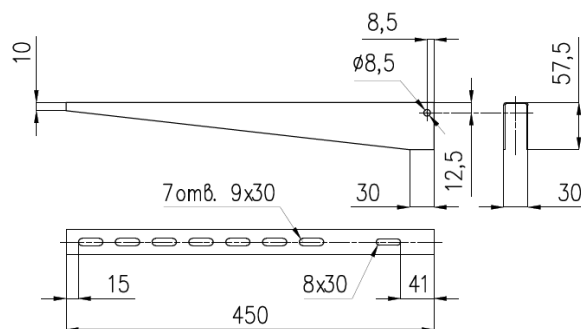
Полка кронштейна КП 400
