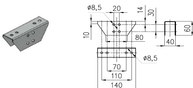
Элемент крепления к потолку сдвоенный КЭП 2
