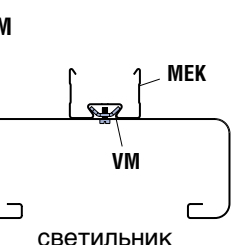
СВЕТИЛЬНИК
