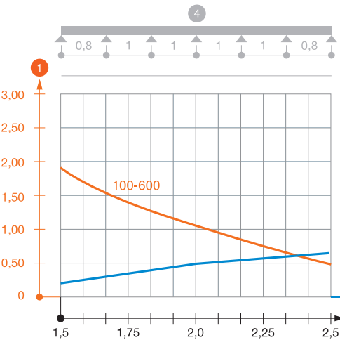
Диаграмма нагрузки на кабельный лоток типа MKSMU 85
