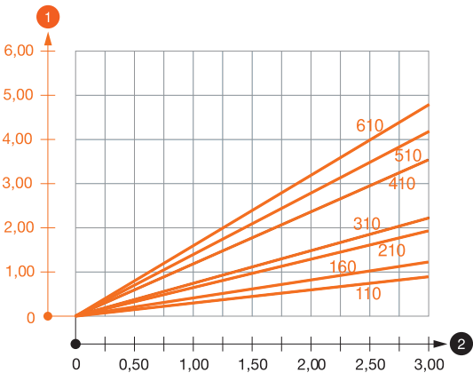
Диаграмма нагрузки на кронштейн AW 30
