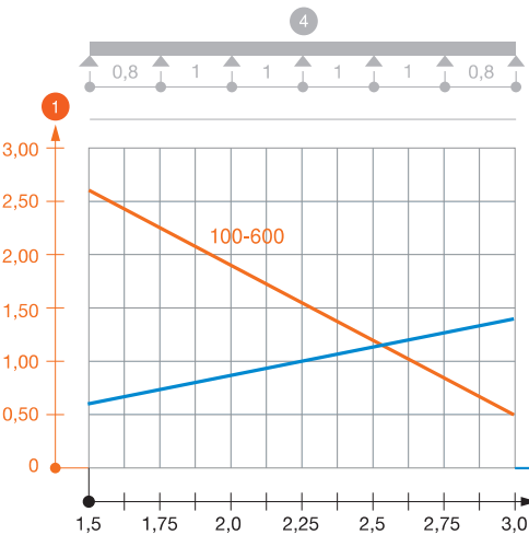
Диаграмма нагрузки на кабельный лоток типа SKSMU 60
