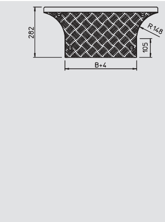
Крышка рифленая для Т-образного / крестового соединения
