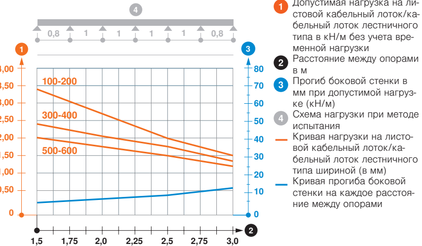
Диаграмма нагрузки на кабельный лоток SKSM 85
