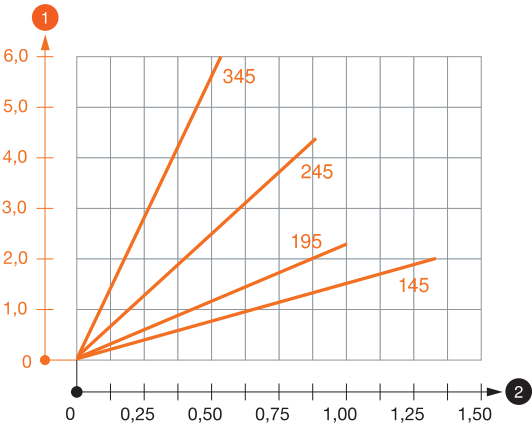
Значения нагрузки на дюбели для TP-кронштейна
