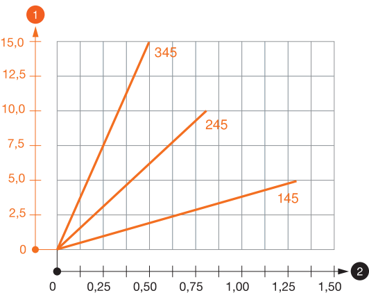
Значения нагрузки на дюбели для настенной / потолочной скобы TPDG
