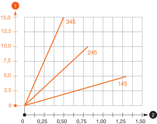
Значения нагрузки на дюбели для настенной / потолочной скобы TPD
