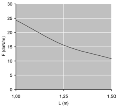
График допустимых нагрузок График действителен для NATO 15, соединенных в один пролет соединителями, удаленными на 1/5 расстояния от точек опоры. Коэффициент запаса прочности - 2. F - максимально допустимая нагрузка (даН/м) L - расстояние между опорами (м) L/200 - деформация при изгибе (м) 1 даН/м = 1 кг/м
